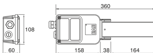
Торцевой питающий элемент
