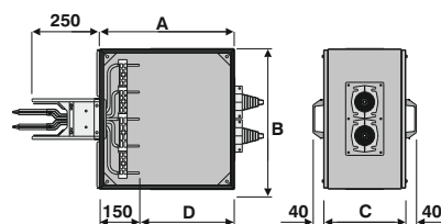
Односторонняя система, 5 проводников
