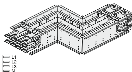
Z-образная горизонтальная вправо
