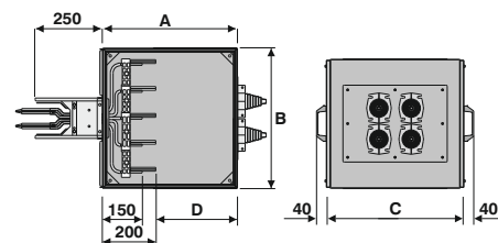
двух- и трехсторонняя система, 5 проводников
